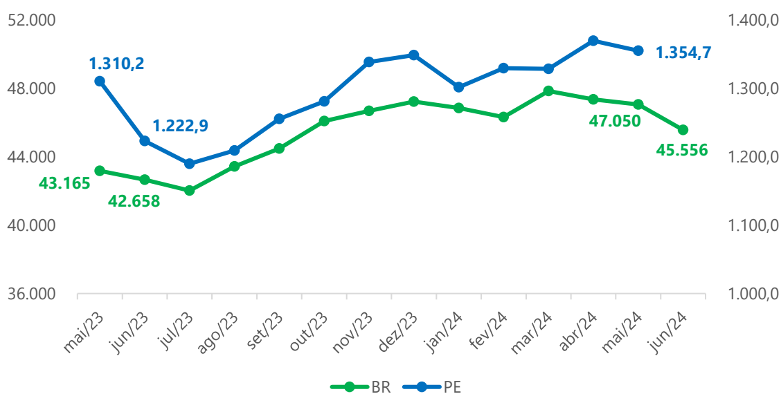
Figura 9 - Consumo de energia elétrica na rede (GWh)
